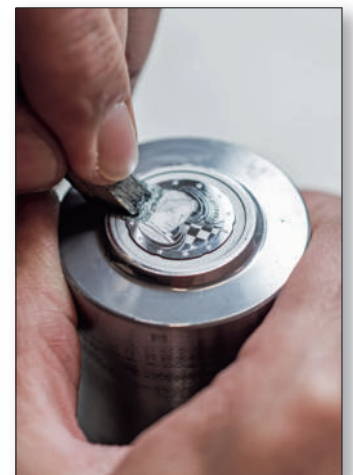
Die Herstellung des „Master Dies“ für Tesla, also des Stempels, von dem alle anderen Stempel abgenommen werden.
