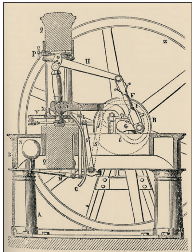
Skizze zur Funktion der Kniehebelpresse.
