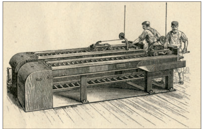
Streckbank, wo der Zain exakt auf die Dicke gebracht wird, die später die Münze haben soll.
