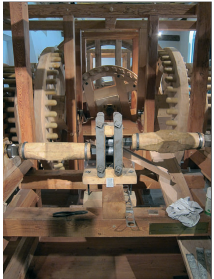
Das nachgebaute Walzprägewerk von Hall. Foto: KW.
